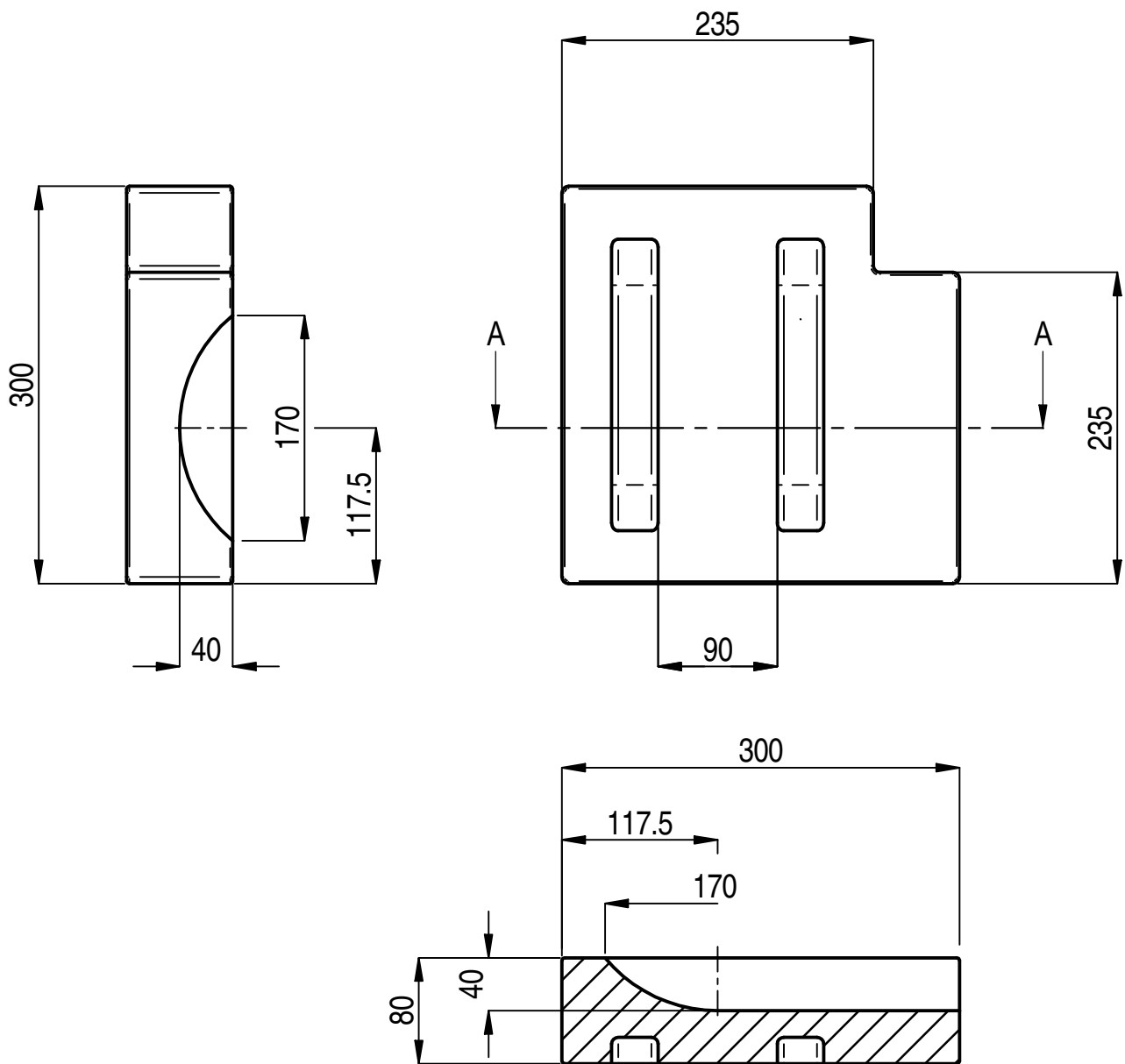
SECTION A-A
